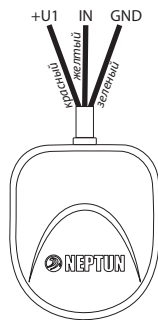
Рис. 7. Маркировка проводов.
